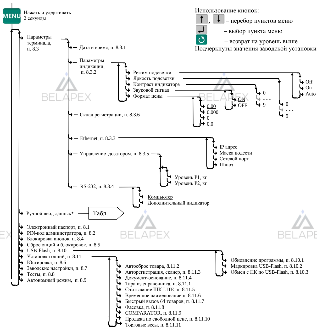
Табл. 8.1 - Структура меню администратора
