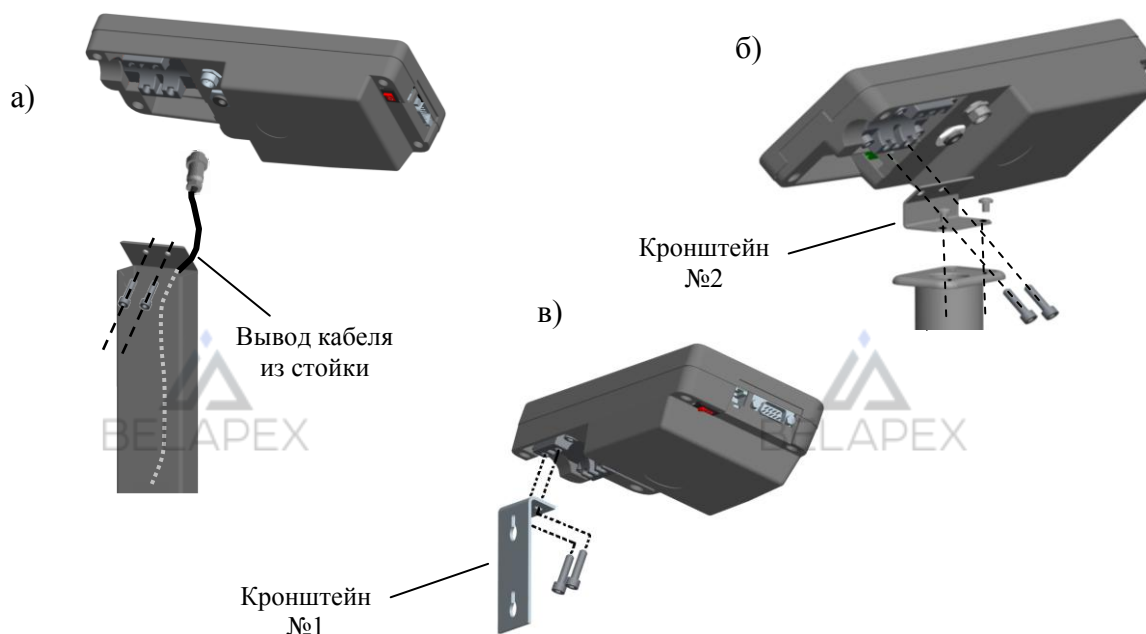
Табл. 2.2 - Варианты крепления терминала RA
